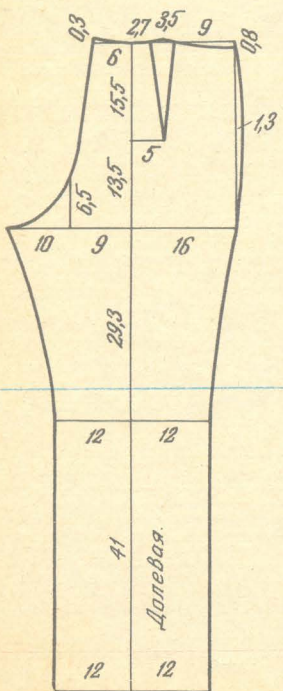
Задняя половинка брюк - 2 дет.
