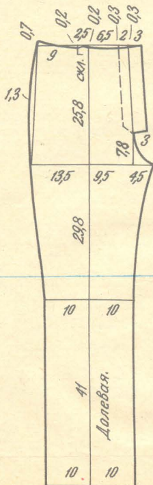
Передняя половинка брюк - 2 дет.
