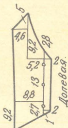
Перед, 2 дет.
