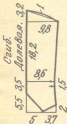
Задняя половинка брюк - 2 дет.
